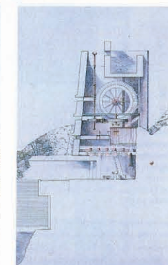
Cyclopentoren, doorsnede.
